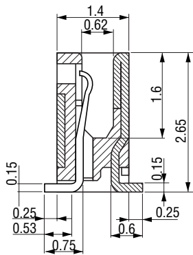
X-X' 断面図
