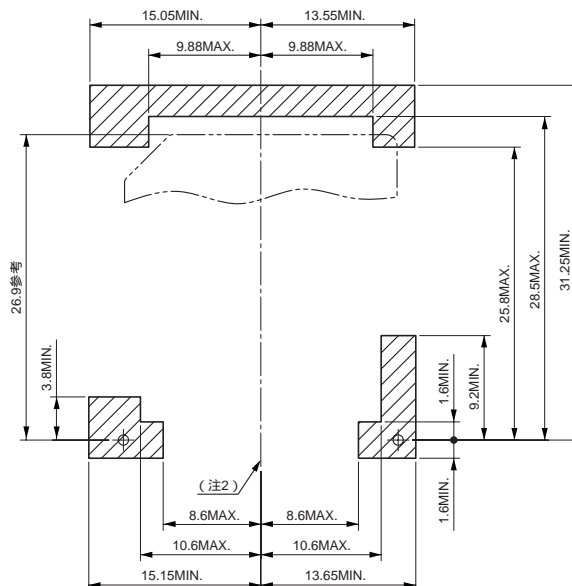
部品搭載不可領域寸法図
